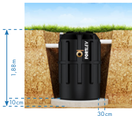
Figura 3 – Instalação sem laje de fechamento.
