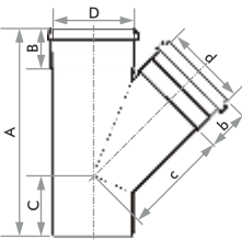
Junção Simples Esgoto SN
