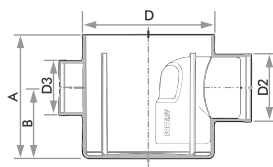
Caixa Sifonada com 3 entradas
