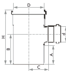
Tê de Redução
