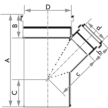
Junção com Redução Esgoto SN
