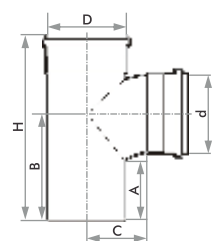
Tê Esgoto
