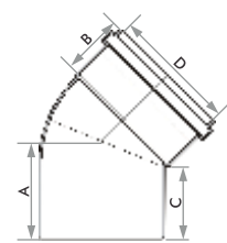
Joelho 45°
