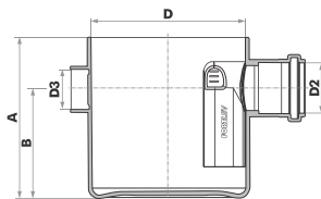
Caixa Sifonada com 7 entradas
