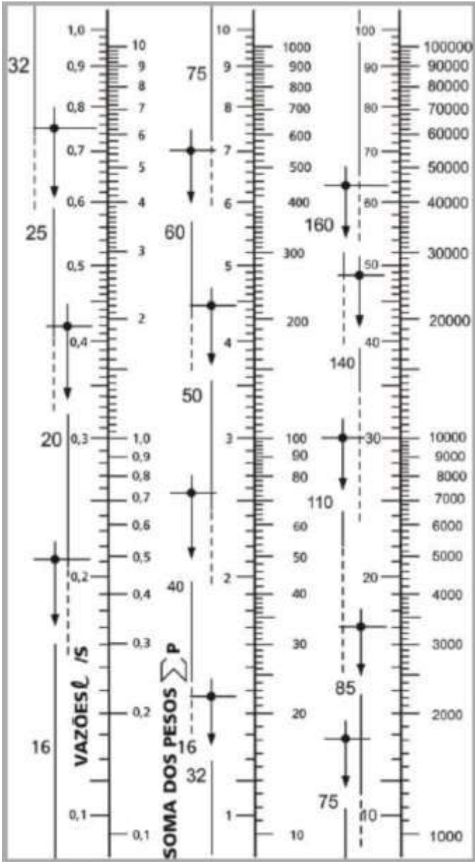
Ábaco 1 - Diâmetros de Tubos de PVC rígido e vazões em função da soma dos pesos
