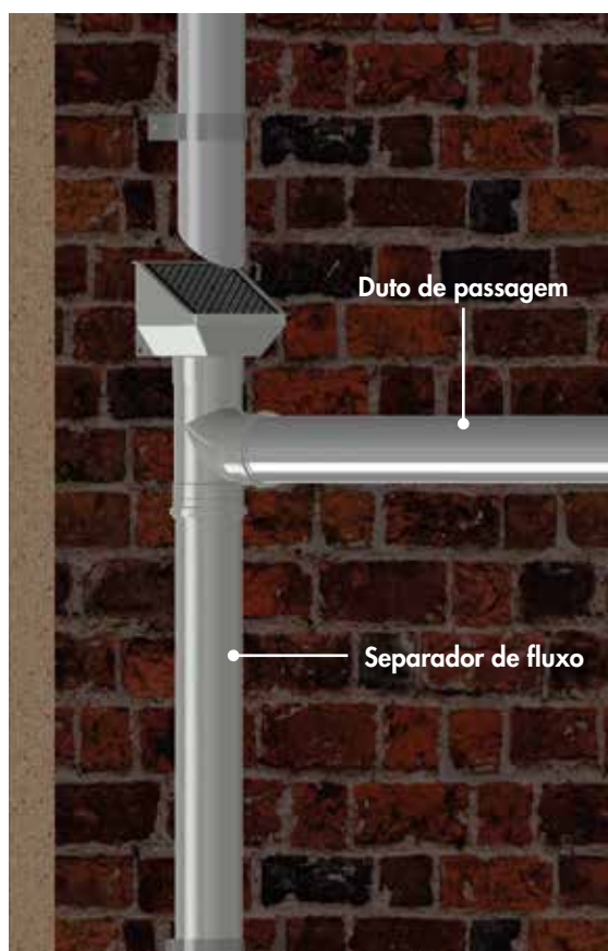
FIG. 09 Saída com derivação para as situações em que houver um separador de fluxo (separador da primeira água de chuva).
